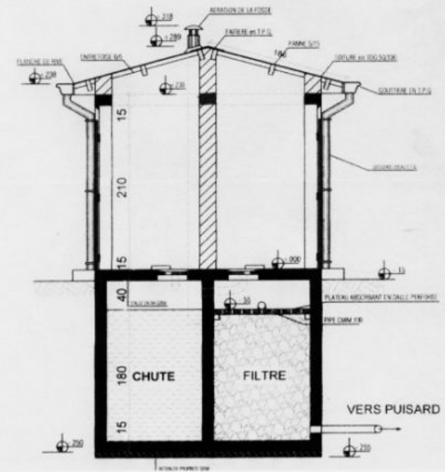
COUPE - AA
